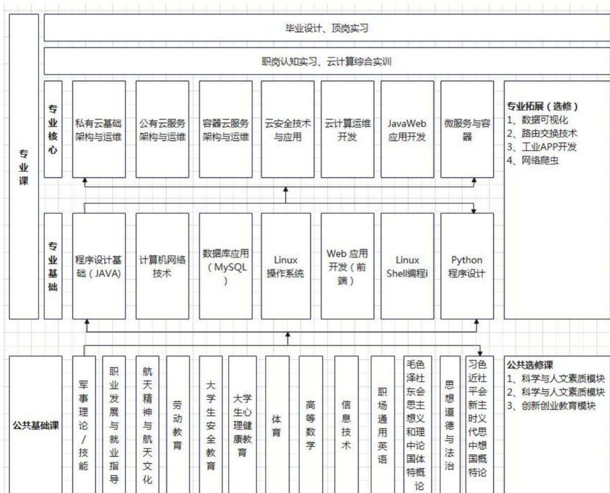
图 1 课程结构图
